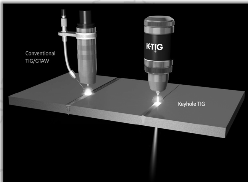
รูปภาพ กระบวนการเชื่อมแบบ Keyhole (K-TIG)
